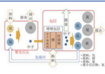
图 8：聚变堆主循环原理示意图
